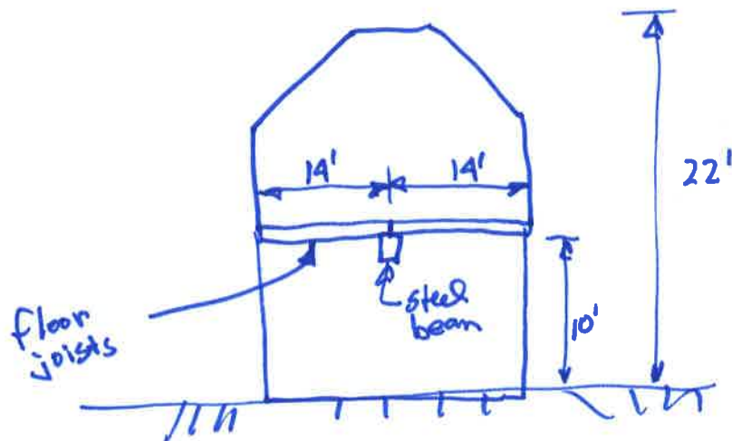
end elevation
